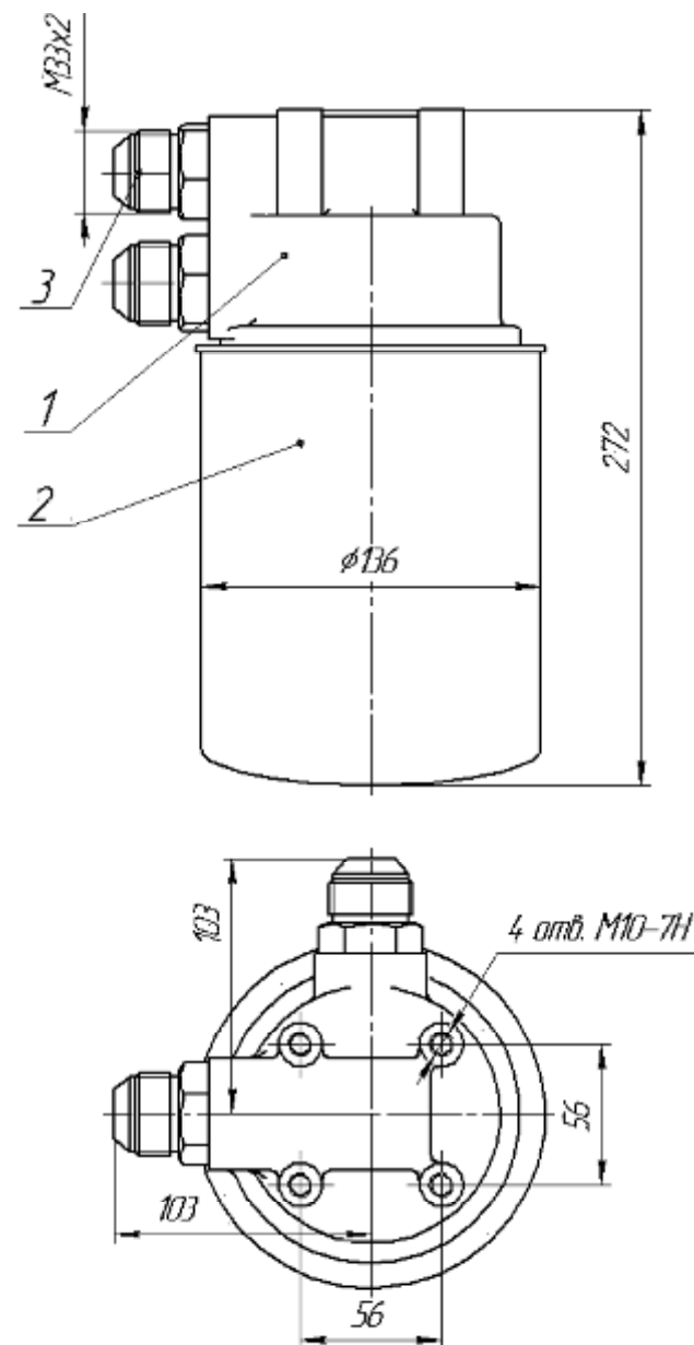
Рисунок 8. Блок распределения.
