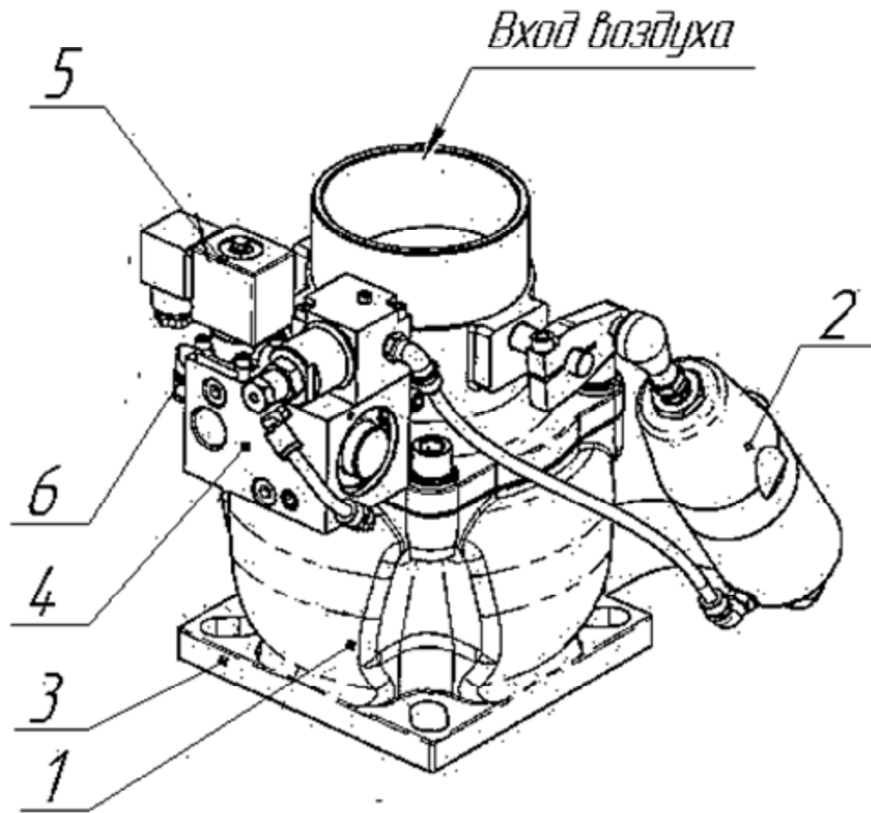
Рисунок 5. Клапан впускной.
